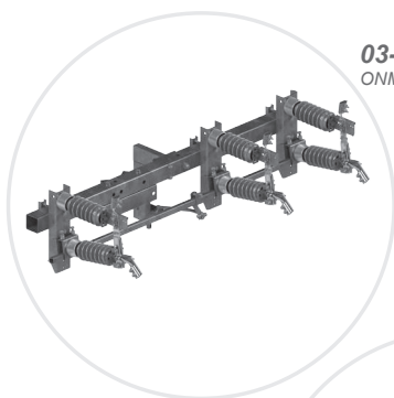
03-021 ONMp III SA 24/4K
