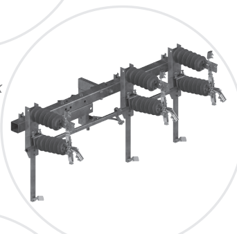
03-026 OUNMp III SA 24/4S
