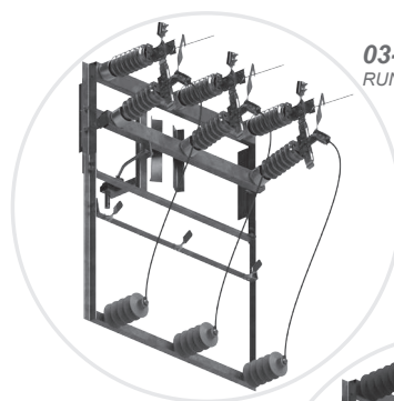
03-040.1 RUNp III SA 24/4Ko
