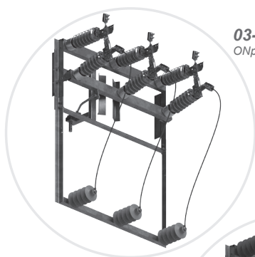
03-037.1 ONp III SA 24/4Ko
