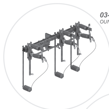
03-082 OUNMp III SA 24/4Ko
