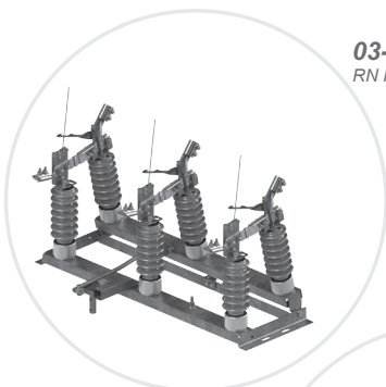
03-007 RN III SA 24/4K
