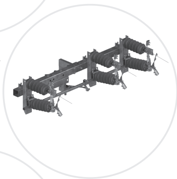
03-027 RNMp III SA 24/4S
