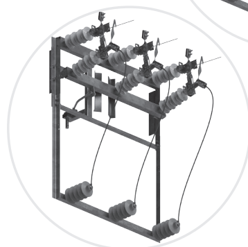
03-043.1 RNp III SA 24/4So
