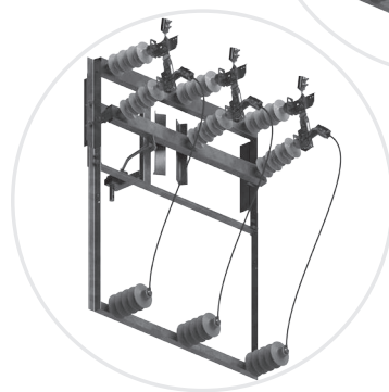
03-041.1 ONp III SA 24/4So
