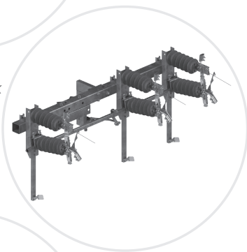
03-028 RUNMp III SA 24/4S
