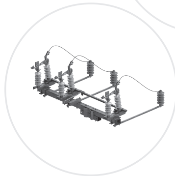
03-073 ONM III SA 24/4So
