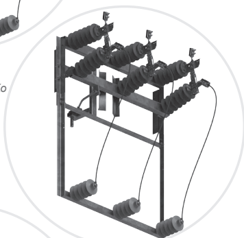
03-041.1 ONp III SA 24/4So
