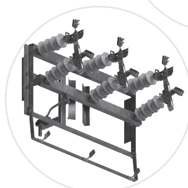
03-042 OUNp III SA 24/4S
