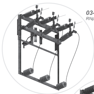
03-039.1 RNp III SA 24/4Ko
