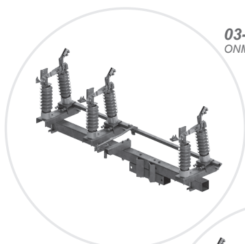
03-053 ONM III SA 24/4K
