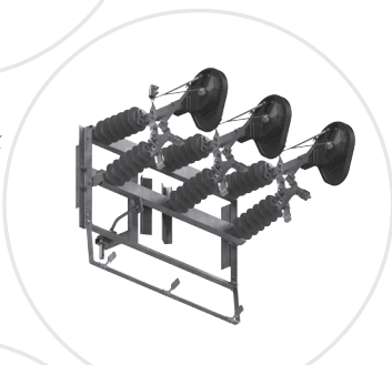
03-744 RUNp III SA 24/4/100S
