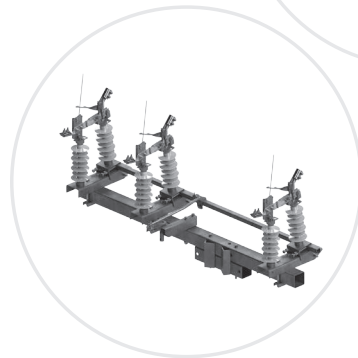
03-059 RNM III SA 24/4S
