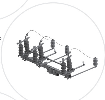
03-074 OUNM III SA 24/4So
