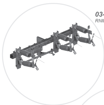
03-023 RNMp III SA 24/4K
