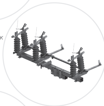
03-060 RUNM III SA 24/4S
