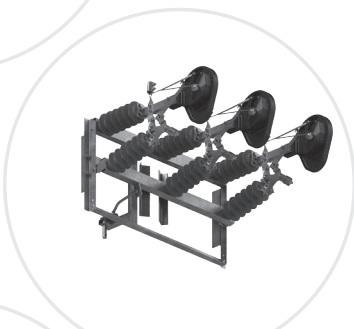
03-743 RNp III SA 24/4/100S
