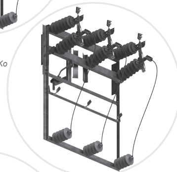
03-042.1 OUNp III SA 24/4So
