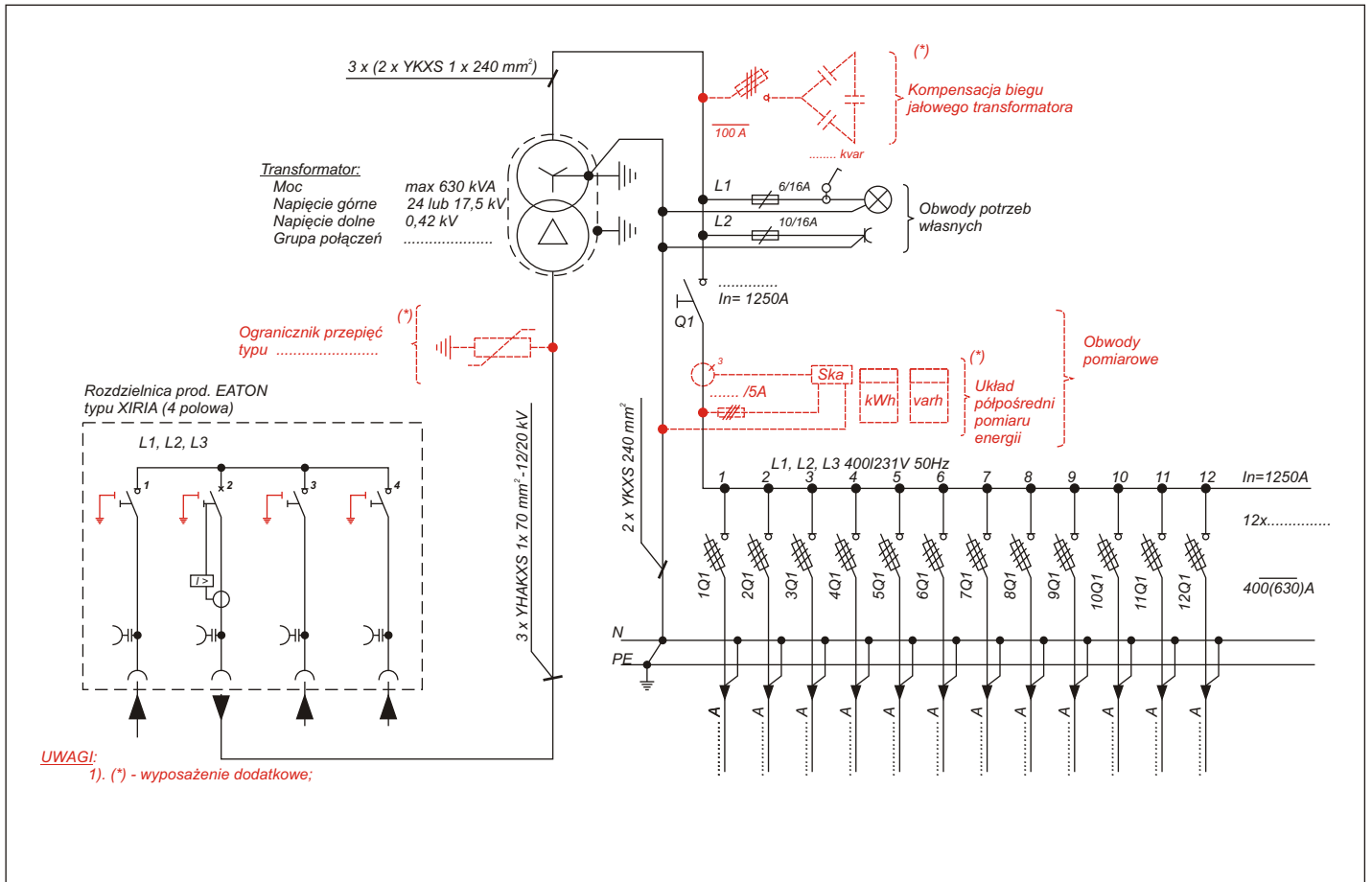
RYS. 5.22. PRZYKŁADOWY SCHEMAT STACJI STLm-2b z ROZDZIELNICĄ TYPU XIRIA PRODUKCJI EATON-Electric.
