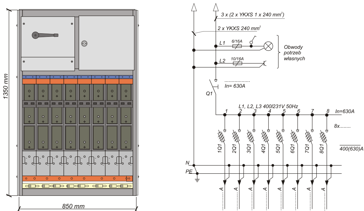
RYS. 5.9. PRZYKŁADOWA ELEWACJA I SCHEMAT ROZDZIELNICYNN W STACJI STLm-1,6b.
