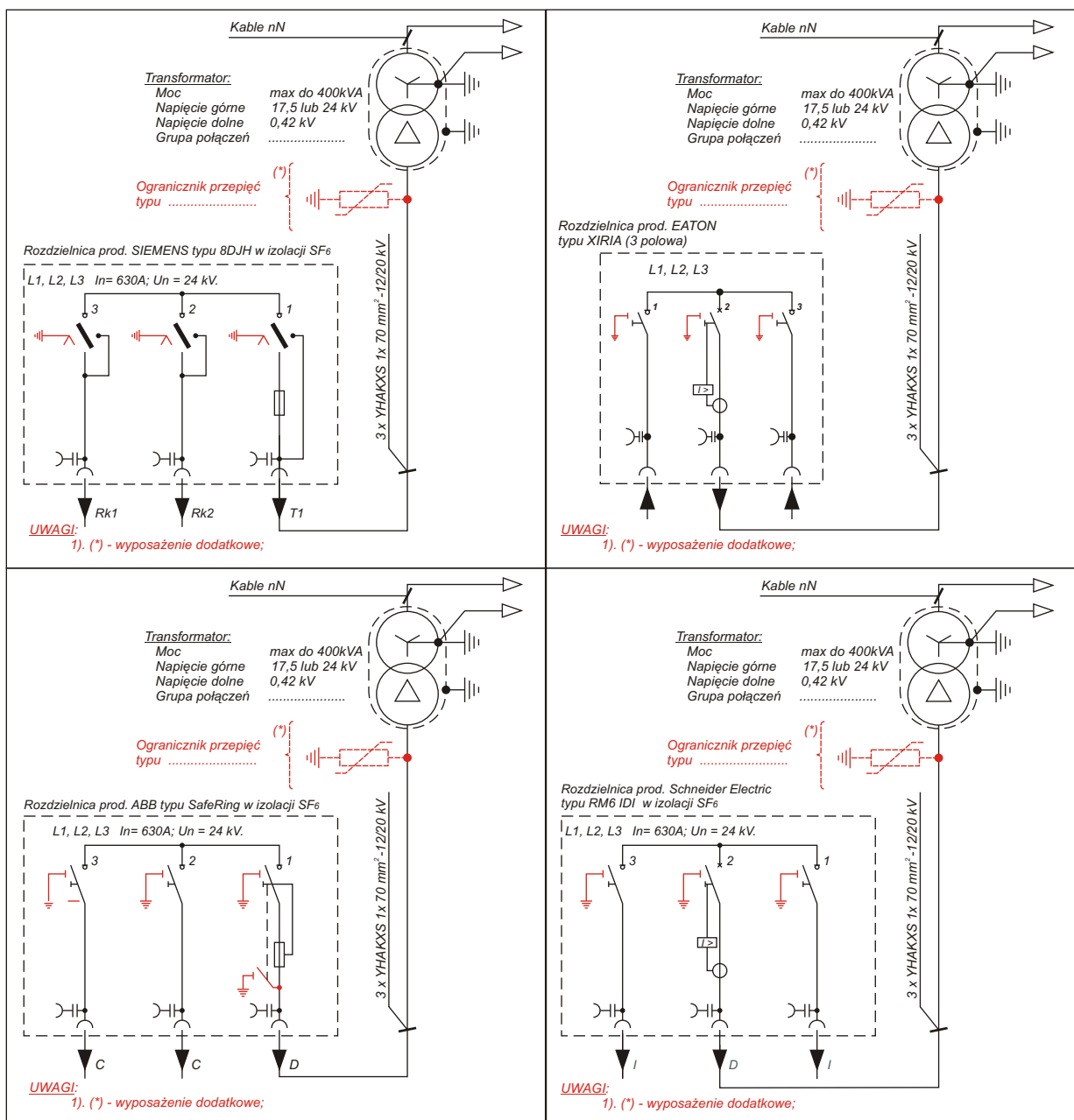
RYS. 5.17. PRZYKŁADOWE SCHEMATY STACJI STLm-1,6b BEZ ROZDZIELNICZY NN.
