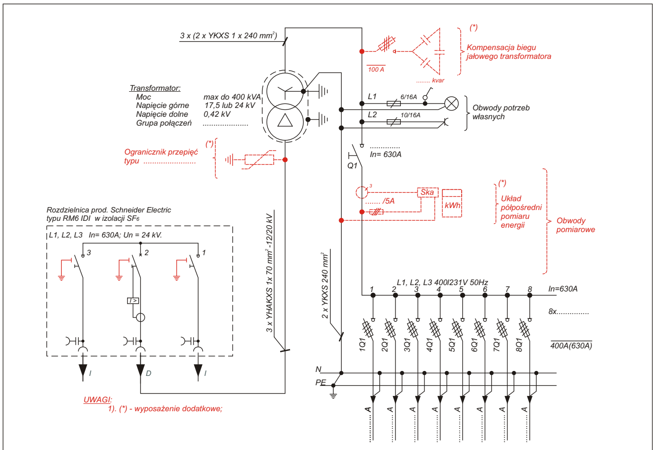
RYS. 5.12. PRZYKŁADOWY SCHEMAT STACJI STLm-1,6b Z ROZDZIELNICĄ TYPU RM6 PRODUKCJI SCHNEIDER ELECTRIC.
