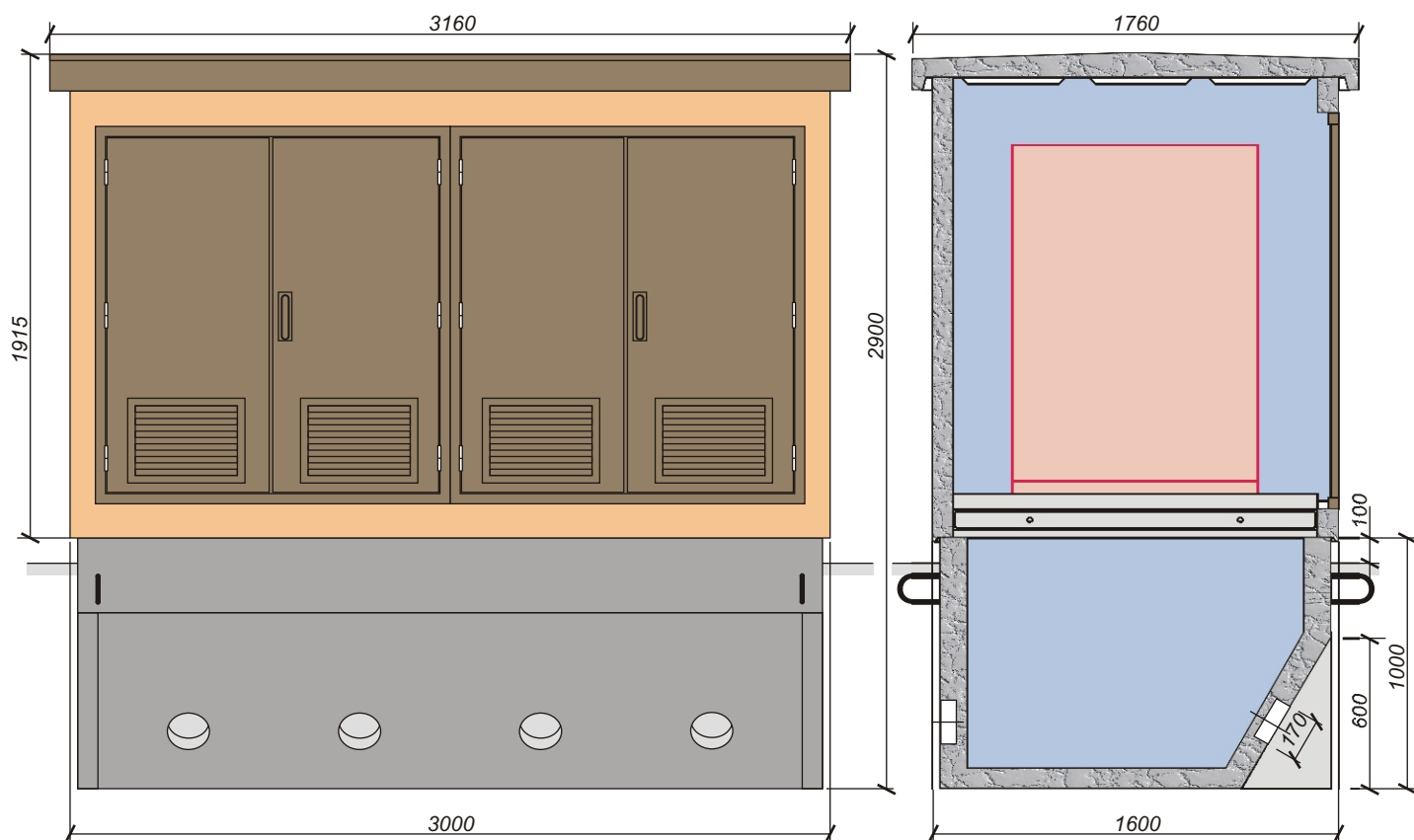
RYS. 12.1. ELEWACJA ZŁĄCZA ZKL-3.
