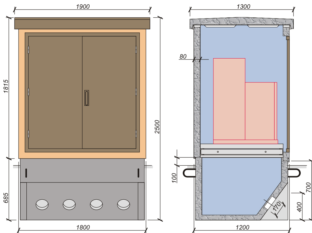
RYS. 12.7. ELEWACJA ZŁĄCZA ZKL-1,8.
